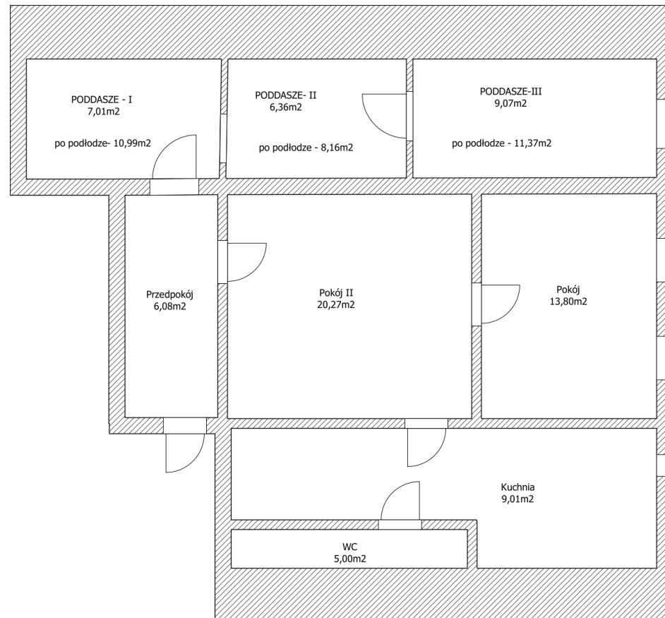
Struktura lokalu do remontu
